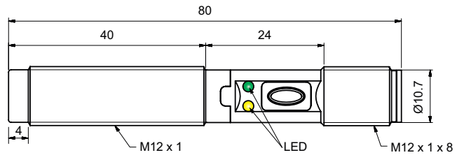
Fig. 5 Plug
